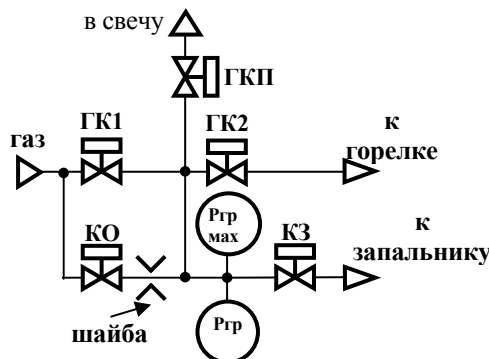
Рисунок Б.2.1 Схема газовой линии, требуемая для реализации алгоритма опрессовки АМАКС
