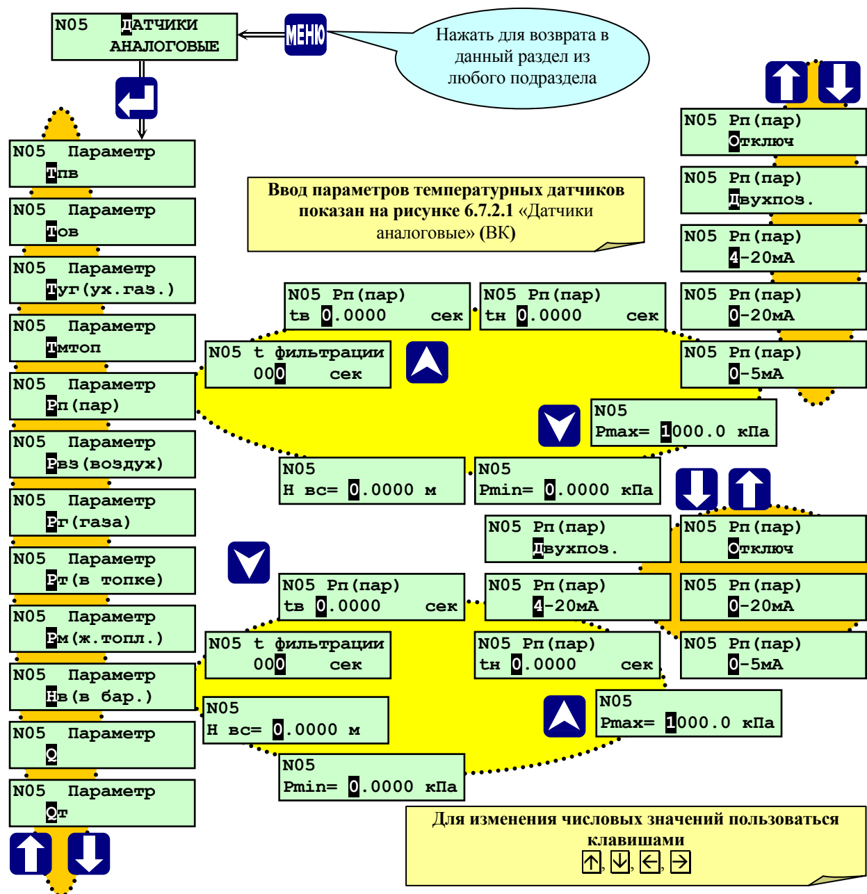
Рисунок 6.7.2.2 Раздел основного меню наладчика «Датчики аналоговые» (паровой котел)
