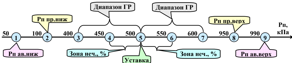
Рисунок 6.8.2.2.1 Соотношение уставок при импульсном и ПИД-регулировании (паровой котел)
