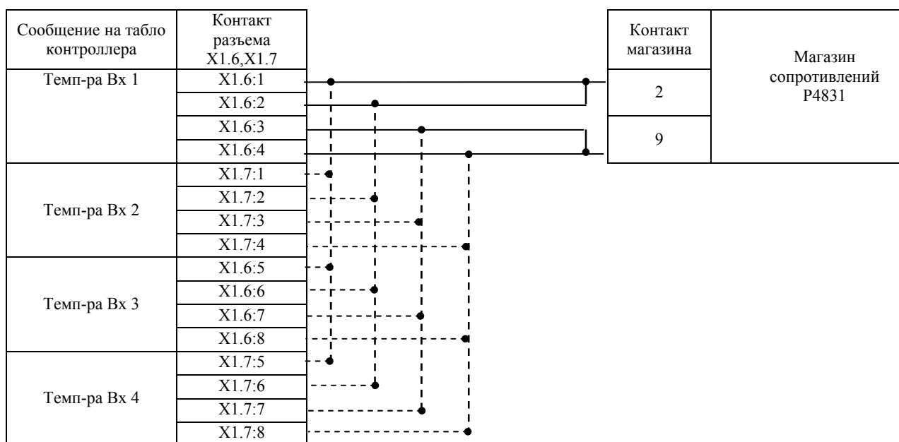
Рисунок Д.2.1 - Схема подключения магазина сопротивлений при настройке IBR, при поверке температурных входов
