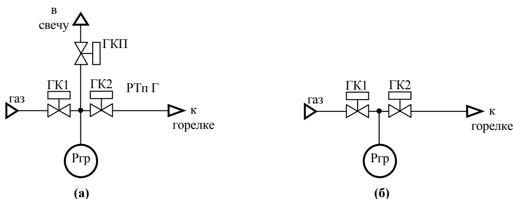
Рисунок Б.1.1 Схемы газовой линии требуемые для реализации алгоритма опрессовки Старорусприбор при наличии (а) и отсутствии (б) продувочной свечи
