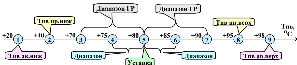
Рисунок 6.8.2.1.1 Соотношение уставок при позиционном регулировании (водогрейный котел)
