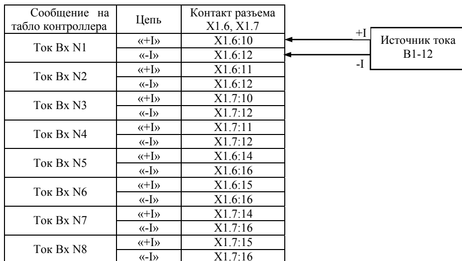
Рисунок Д.2.2 - Схема подключения источника тока при настройке ИВІ, при поверке токовых входов
