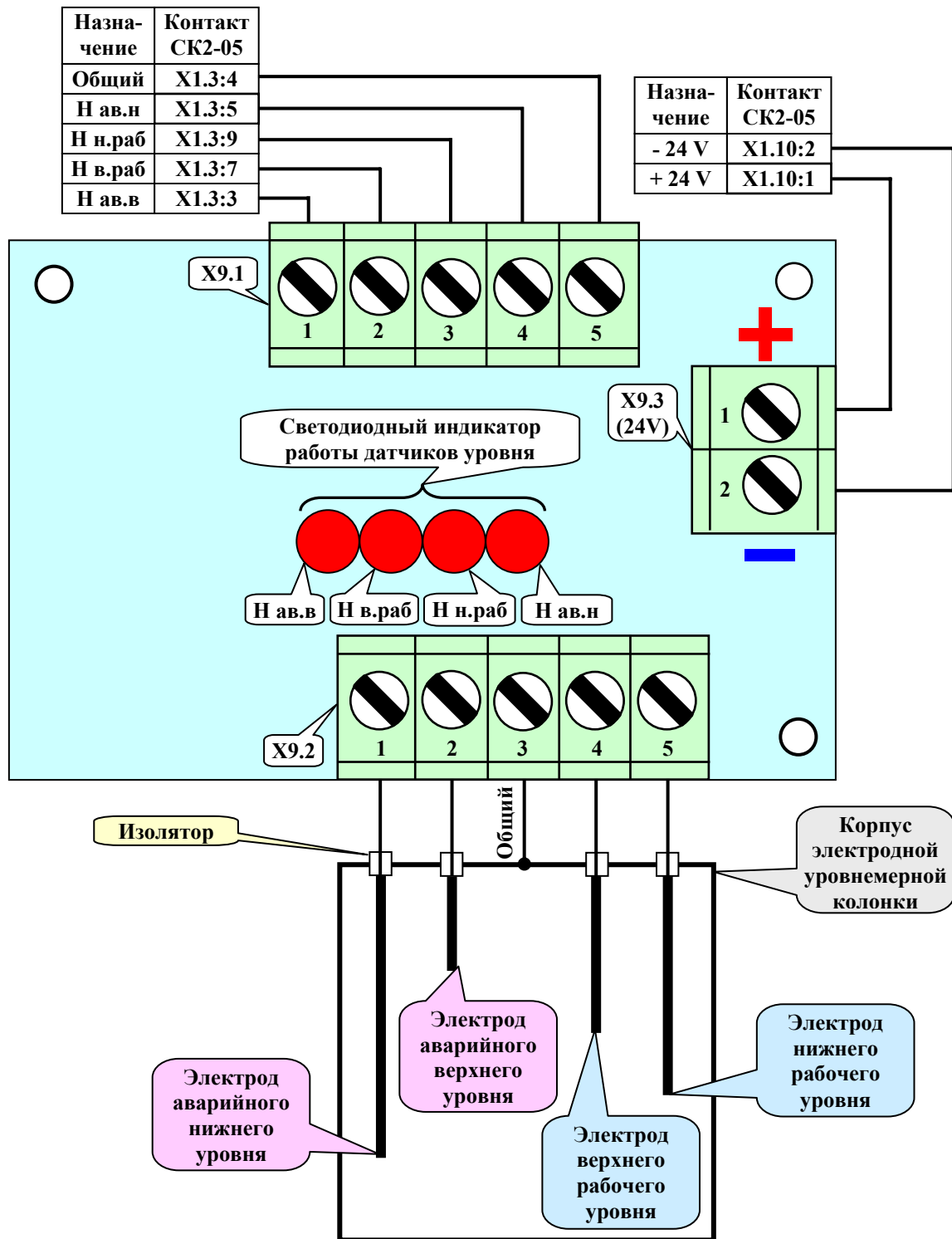
Рисунок А.2.1.7 - Подключение платы УК (уровнемерной колонки) и нумерация её разъёмов
