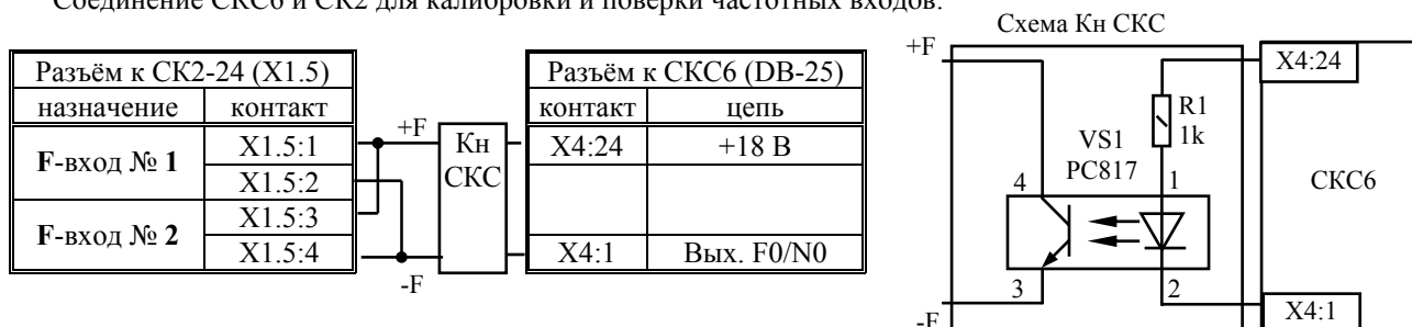
Рисунок Д.3.2 - Распайка разъемов к СКС6 и подключение к разъемам СК1-24 для подключения частотных сигналов
