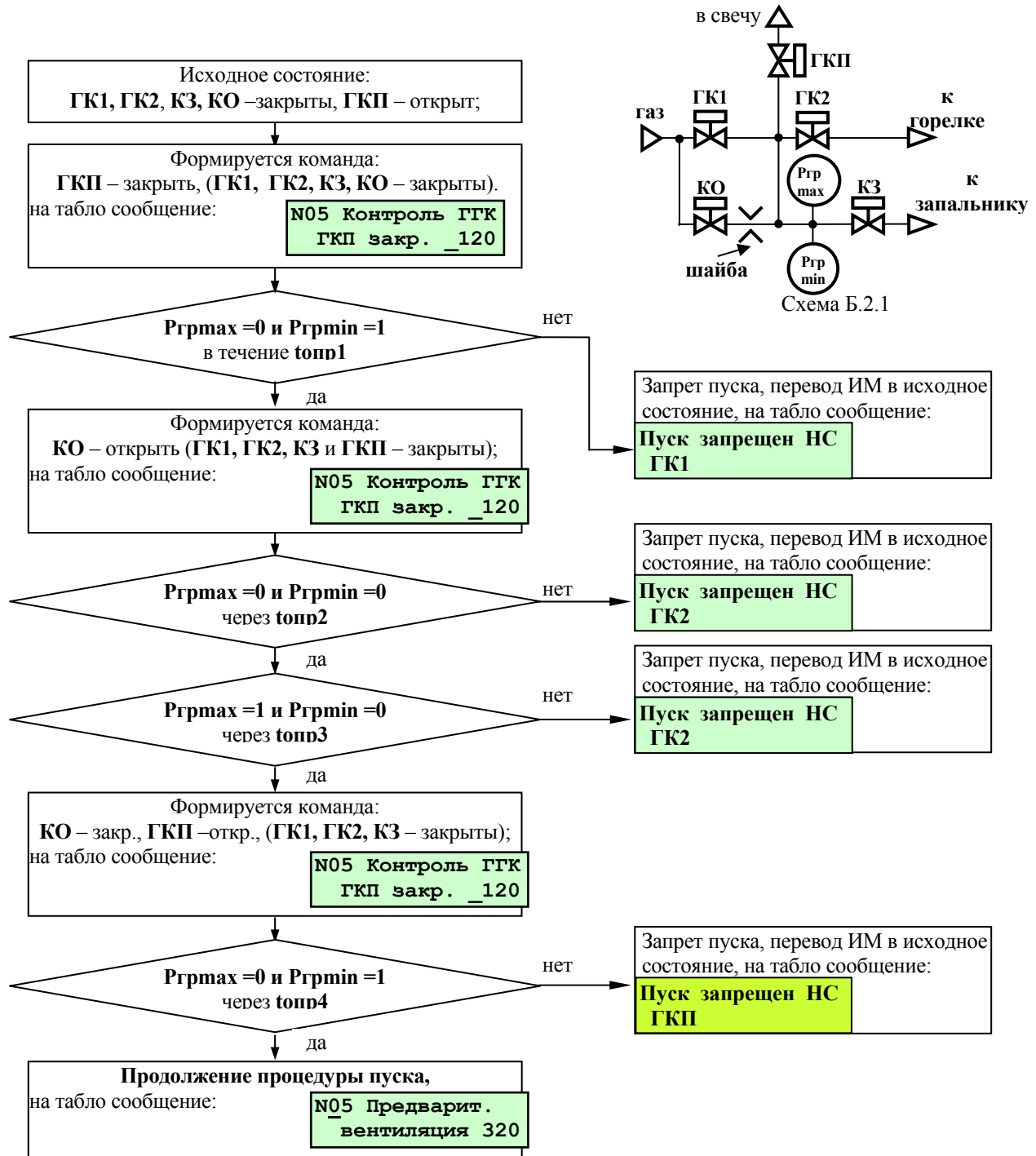
Рисунок Б.2.2 Блок-схема алгоритма опрессовки «АМАКС» для схемы газовой линии, приведенной на рисунке Б.2.1.
