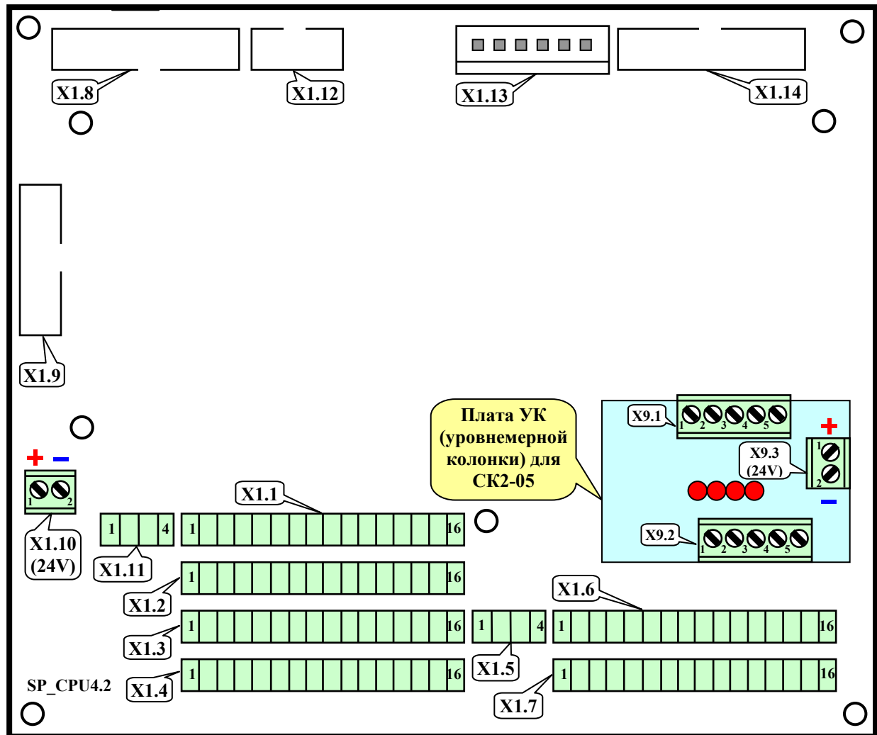
Рисунок А.2.1.1 - Расположение разъёмов на системной плате SP_CPU и их нумерация, размещение платы УК (уровнемерной колонки) и нумерация её разъёмов
