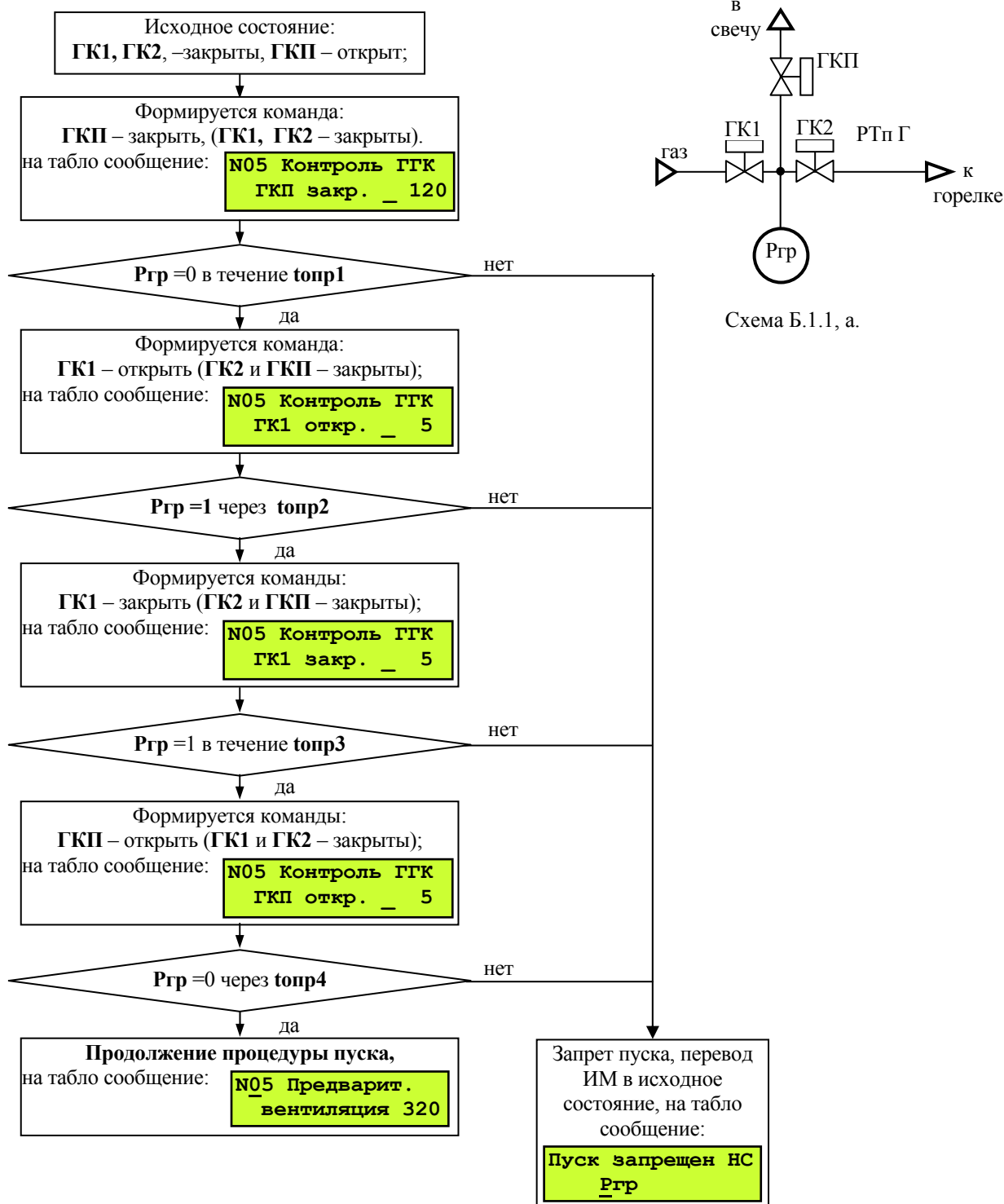
Рисунок Б.1.2 Блок-схема алгоритма опрессовки «Старорусприбор» для схемы газовой линии, приведенной на рисунке Б.1.1, а.
