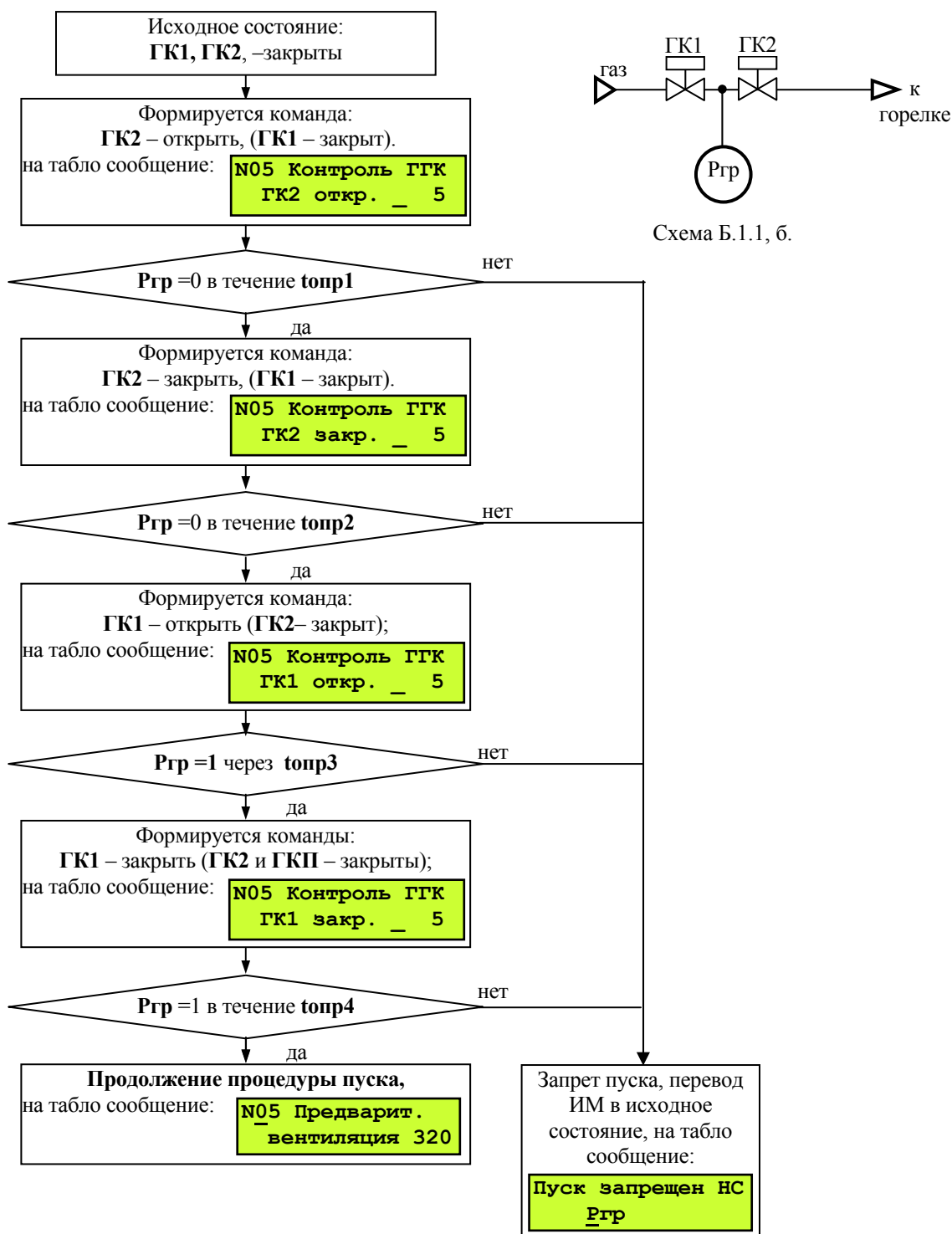
Рисунок Б.1.3 Блок-схема алгоритма опрессовки «Старорусприбор» для схемы газовой линии, приведенной на рисунке Б.1.1, б
