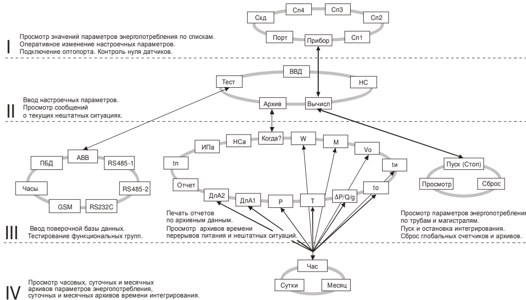
Рисунок 5.1 – Структура меню
