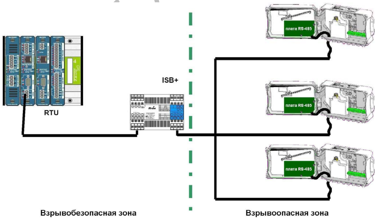
Рис. 3. Многоточечное соединение корректоров по интерфейсу RS-485
