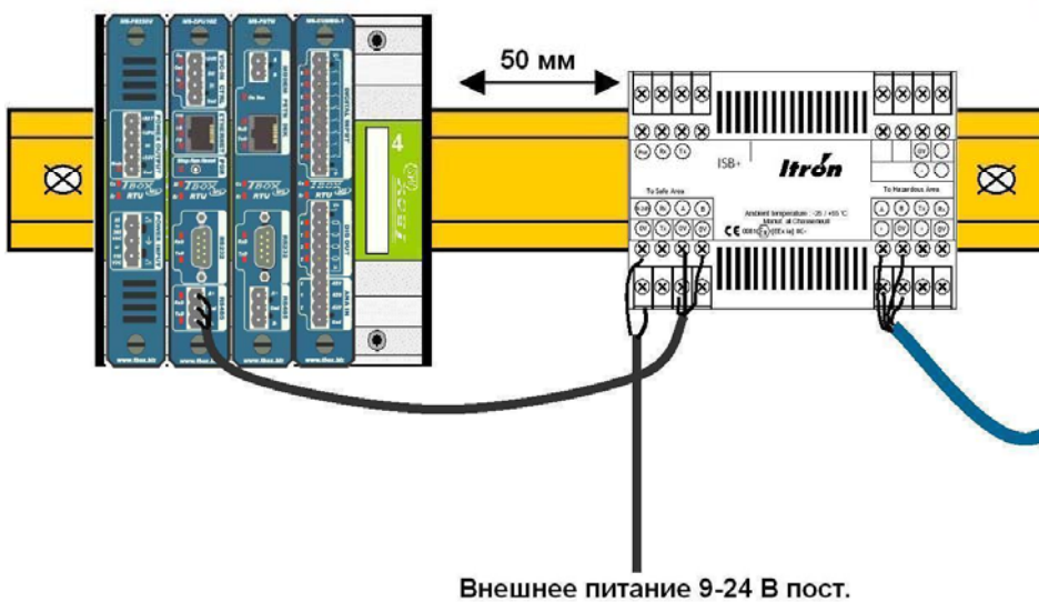
Рис. 4. Сбор данных по интерфейсу RS-485
